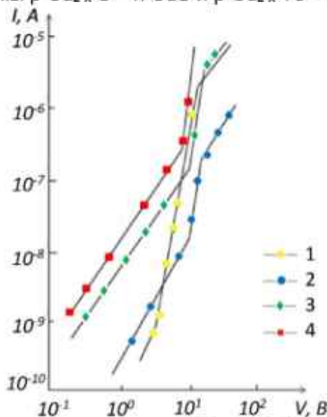
Рис.2. Обратные ветви BAX гетероперехода p CdTe – n CdS при различных температурах, К: 1-302, 2-338, 3-358, 4-376
