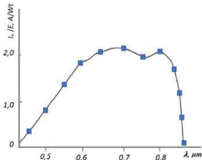
Рис. 3. Спектральное распределение фоточувствительности структуры p CdTe – n CdSe
