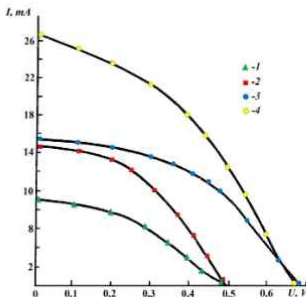
Рис.1. Нагрузочная BAX пленочной структуры p CdTe – n CdS (3,4) и p CdTe – n CdSe (1,2) при освещении W – лампой накаливания (1,3) и источником внеатмосферного солнца (2,4) с мощностью 55 и 139 \frac{\text{мВт}}{\text{см}^2} .
