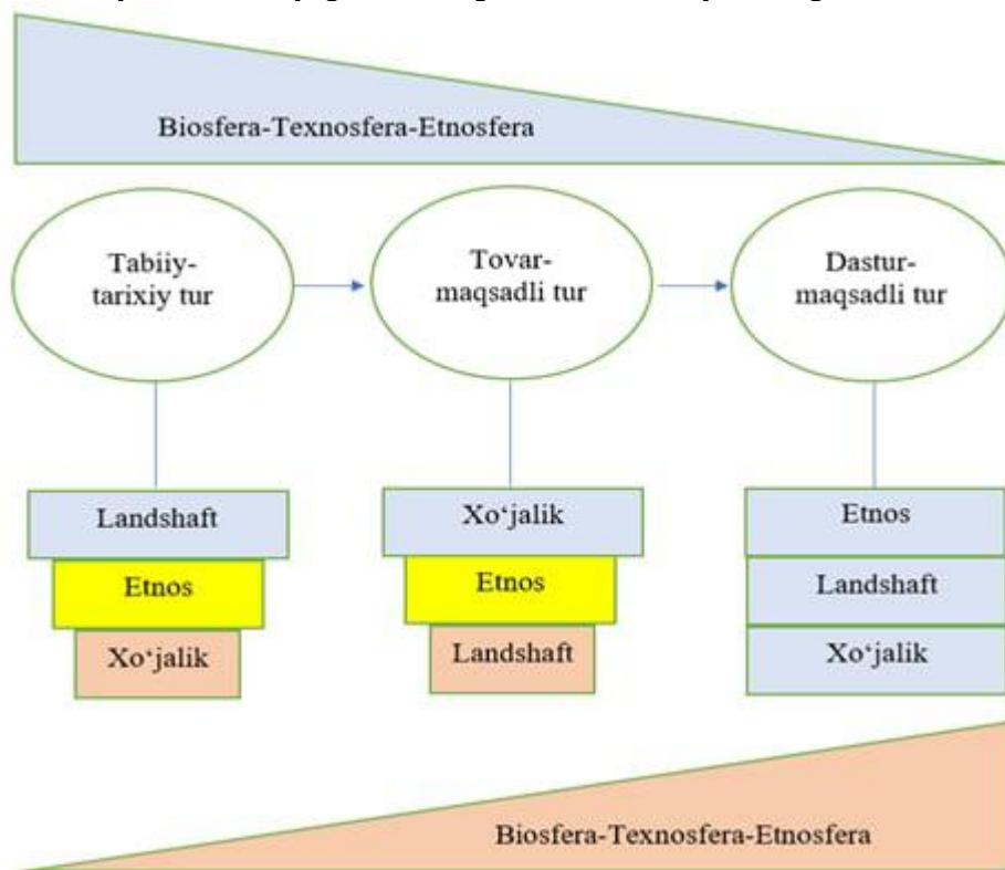
1-rasm. Tabiatdan foydalanishda «landshaft-etnos-xo'jalik» tizimining o'zgarishi
