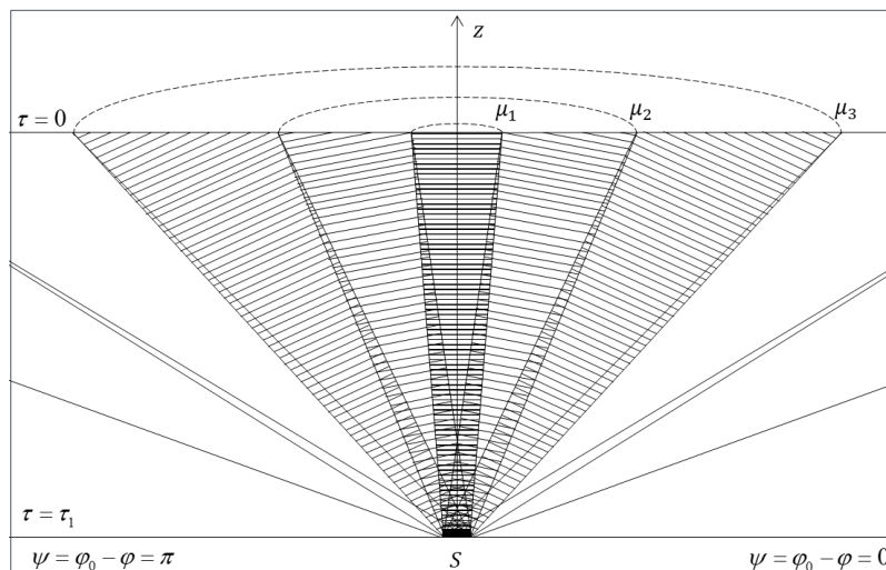
1-rasm. Yer sirtining birlik yuzasidan qaytgan oqimni atmosferada turli yo'nalishlarida taqsimlanishi.
